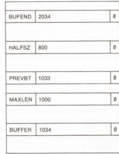
5 BUFEND EQU *
