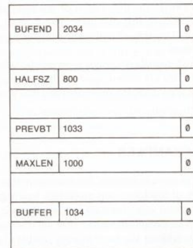
5 BUFEND EQU *
